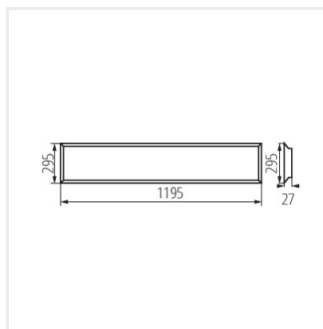
BLINGO 34W 4080 120NW
