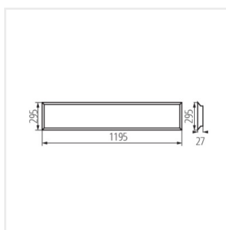
BLINGO 38W 4560 120NW
