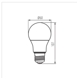
IQ-LED A60 5,9W-CW
